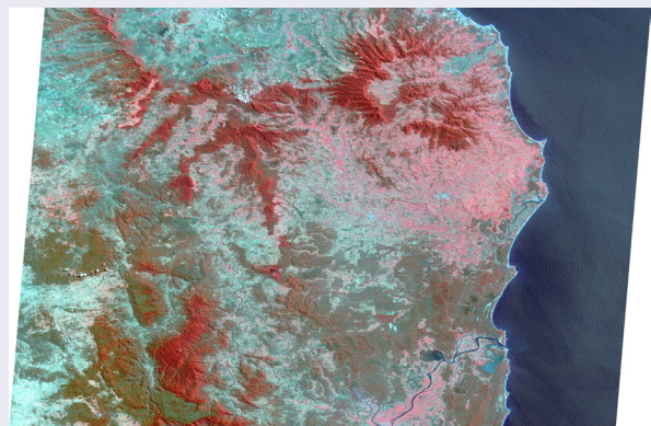
b. Path 89 Row 80
