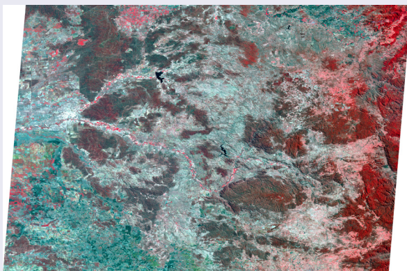
a. Path 90 Row 80
